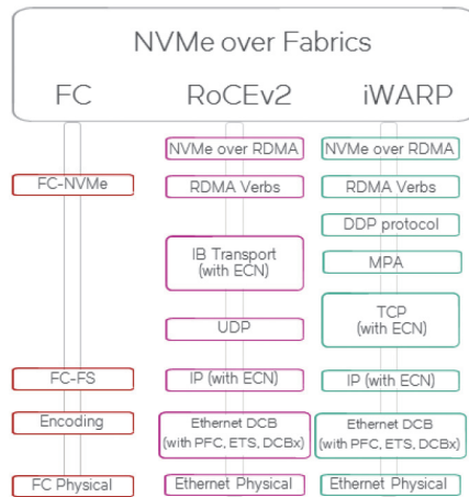
Рис. 4. Сравнение стека для различных NVMe фабрик.
