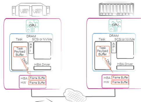
Рис. 2. Fibre Channel выполняет нулевое копирование.
